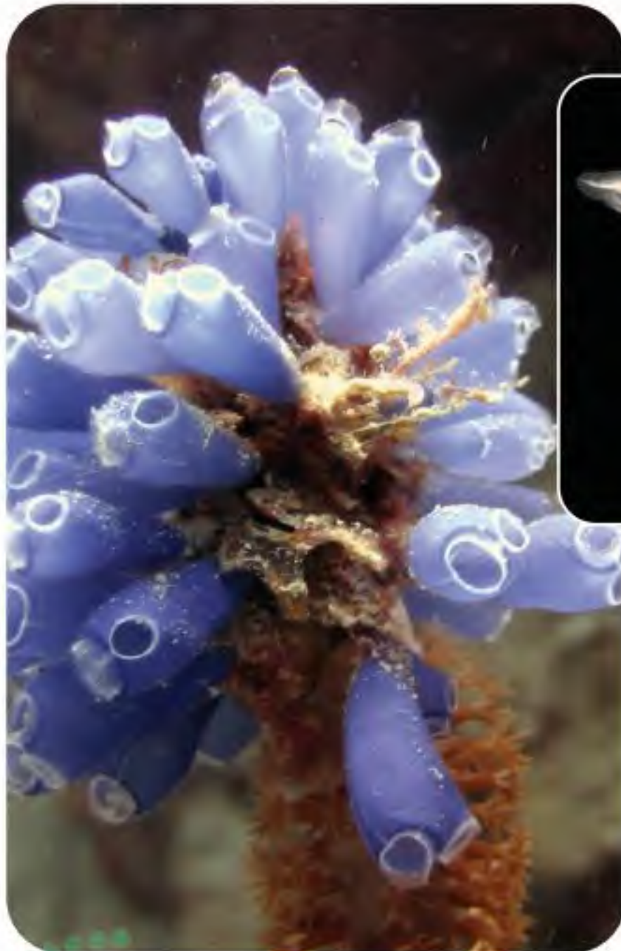
الكيسيات (Tunicate)
