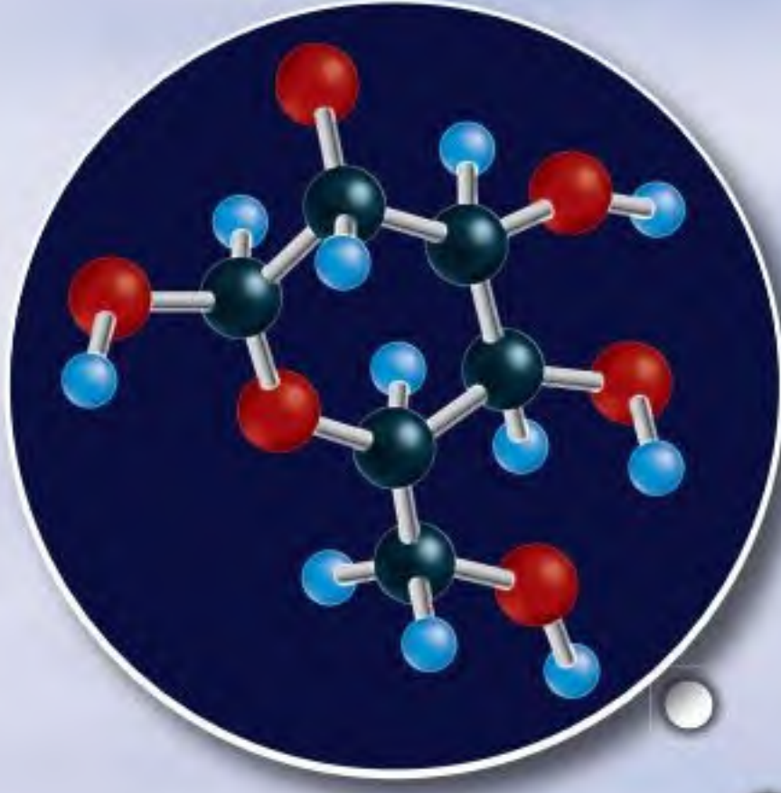
الجلوكوز
