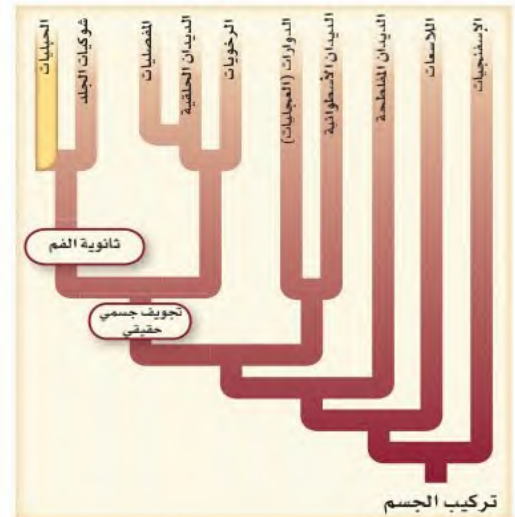
السهيم (Lancelet)
