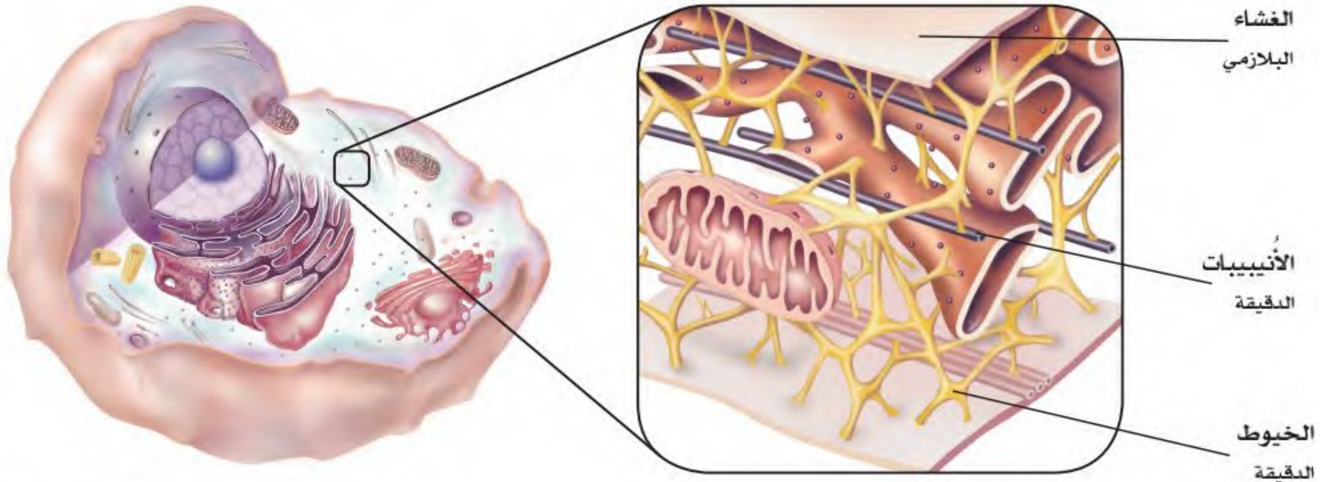
الهيكل الخلوي
