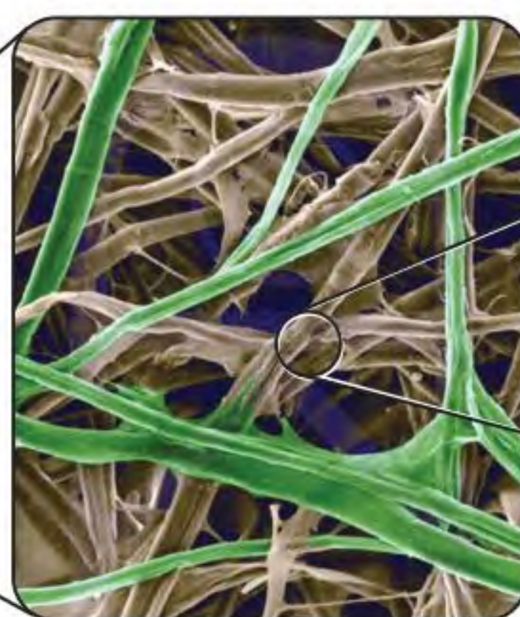
ألياف سيليلوز
