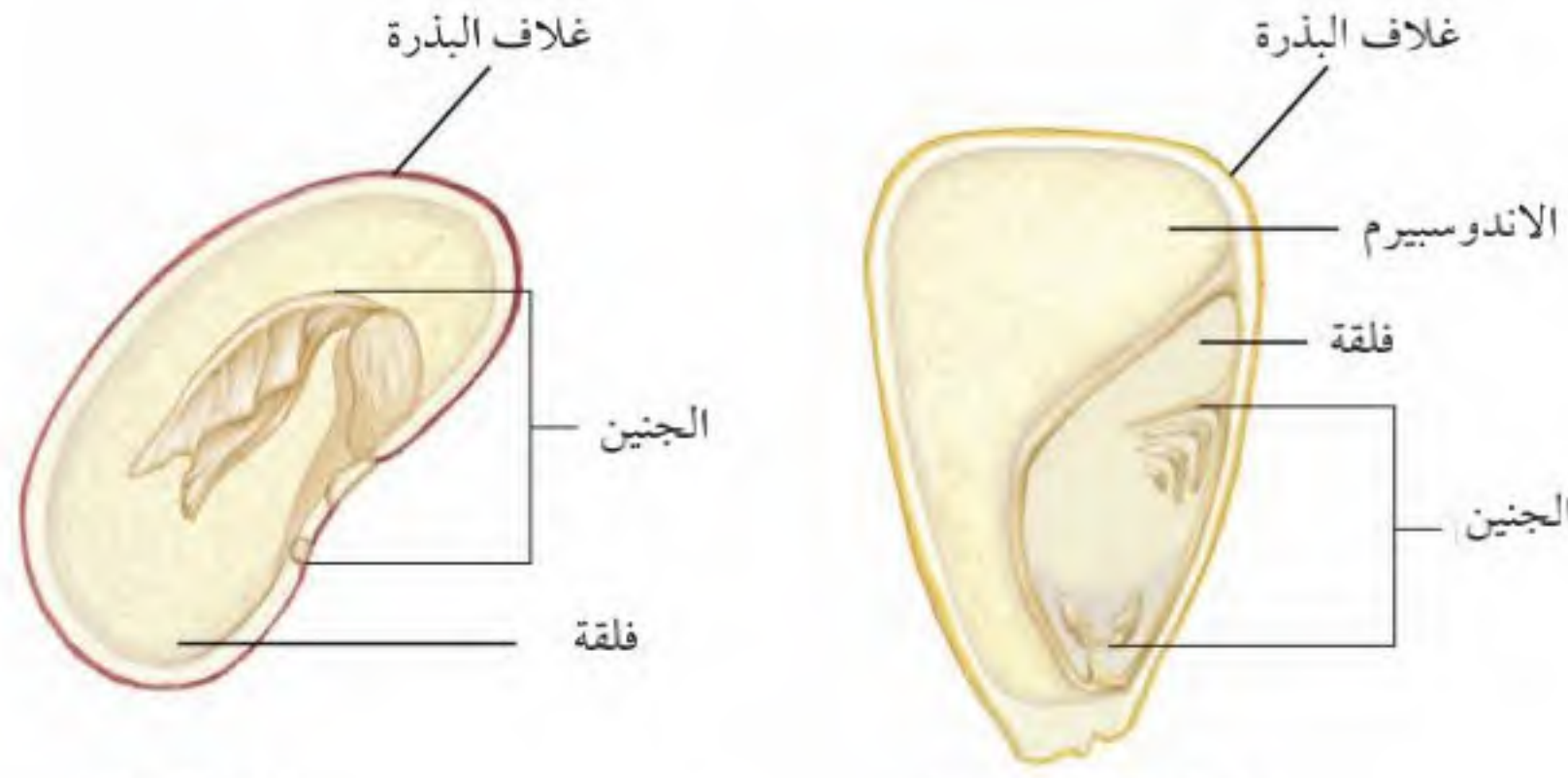
ذوات الفلقتين
