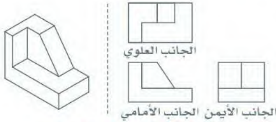
شكل 2.18: أمثلة على الإسقاط المتعامد
