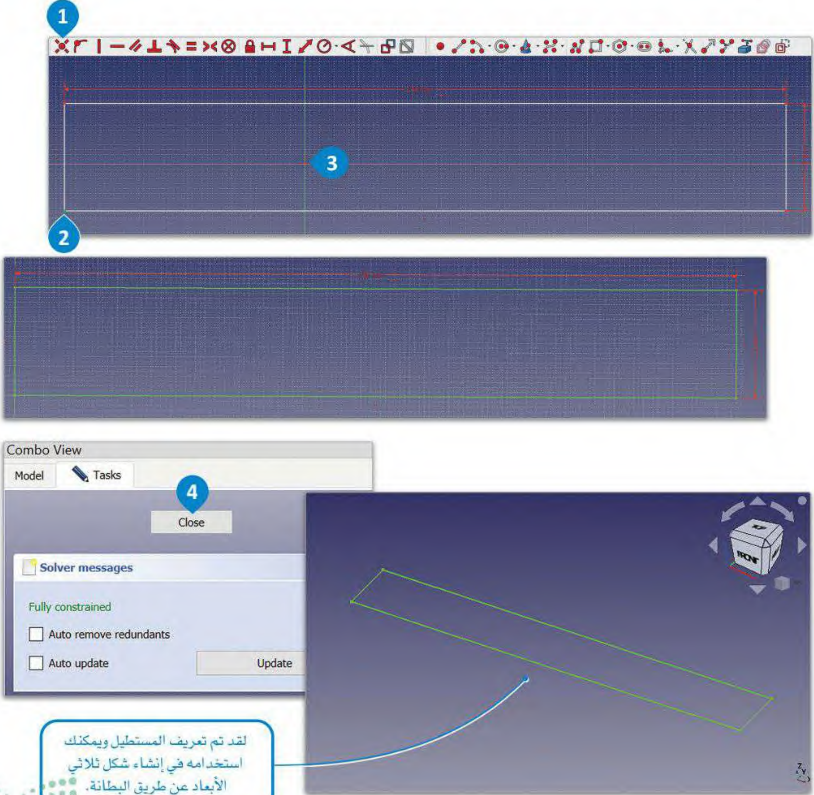
شكل 3.45: تقييد النقاط
