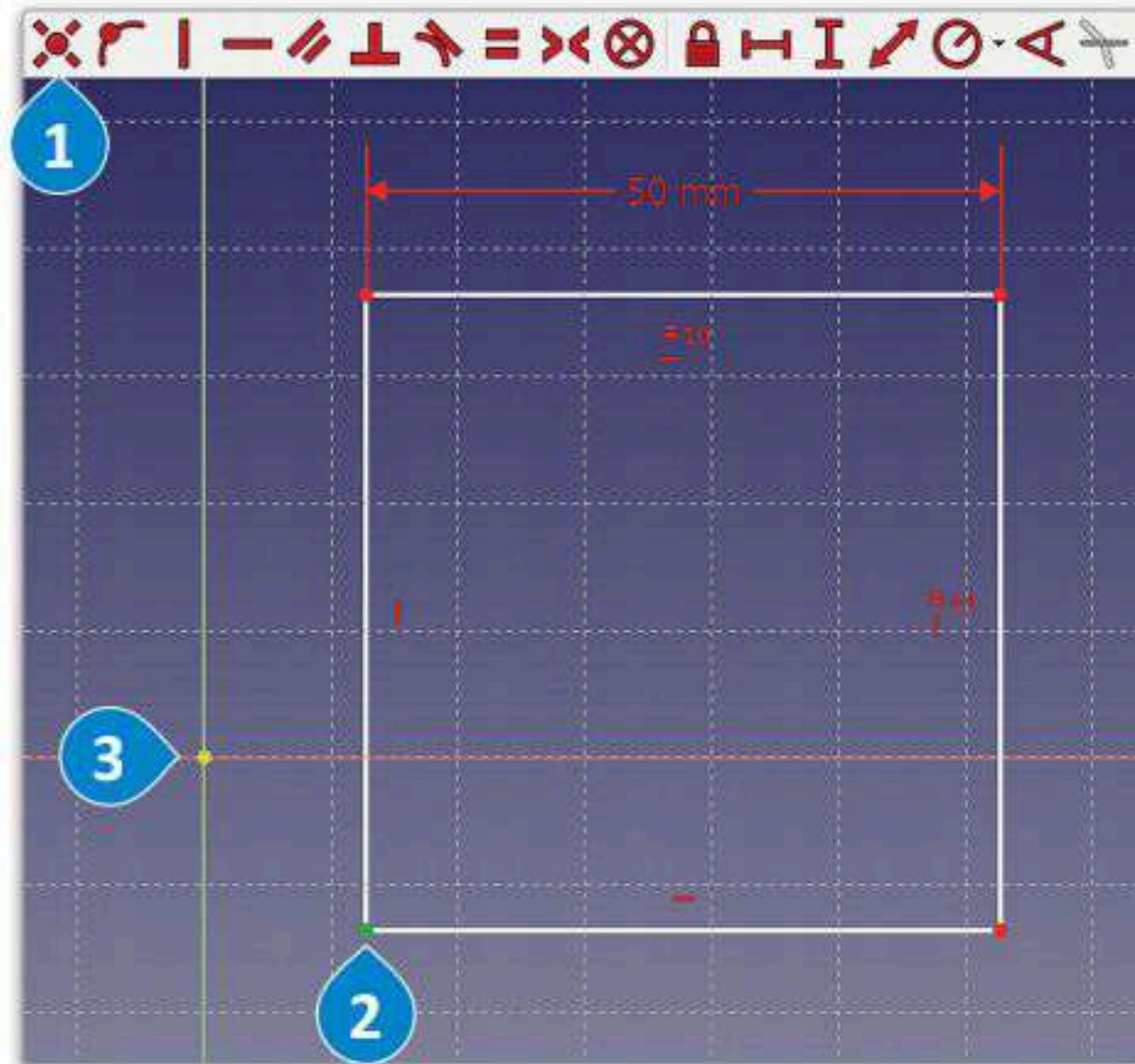
شكل 2.36: تقييد النقاط
