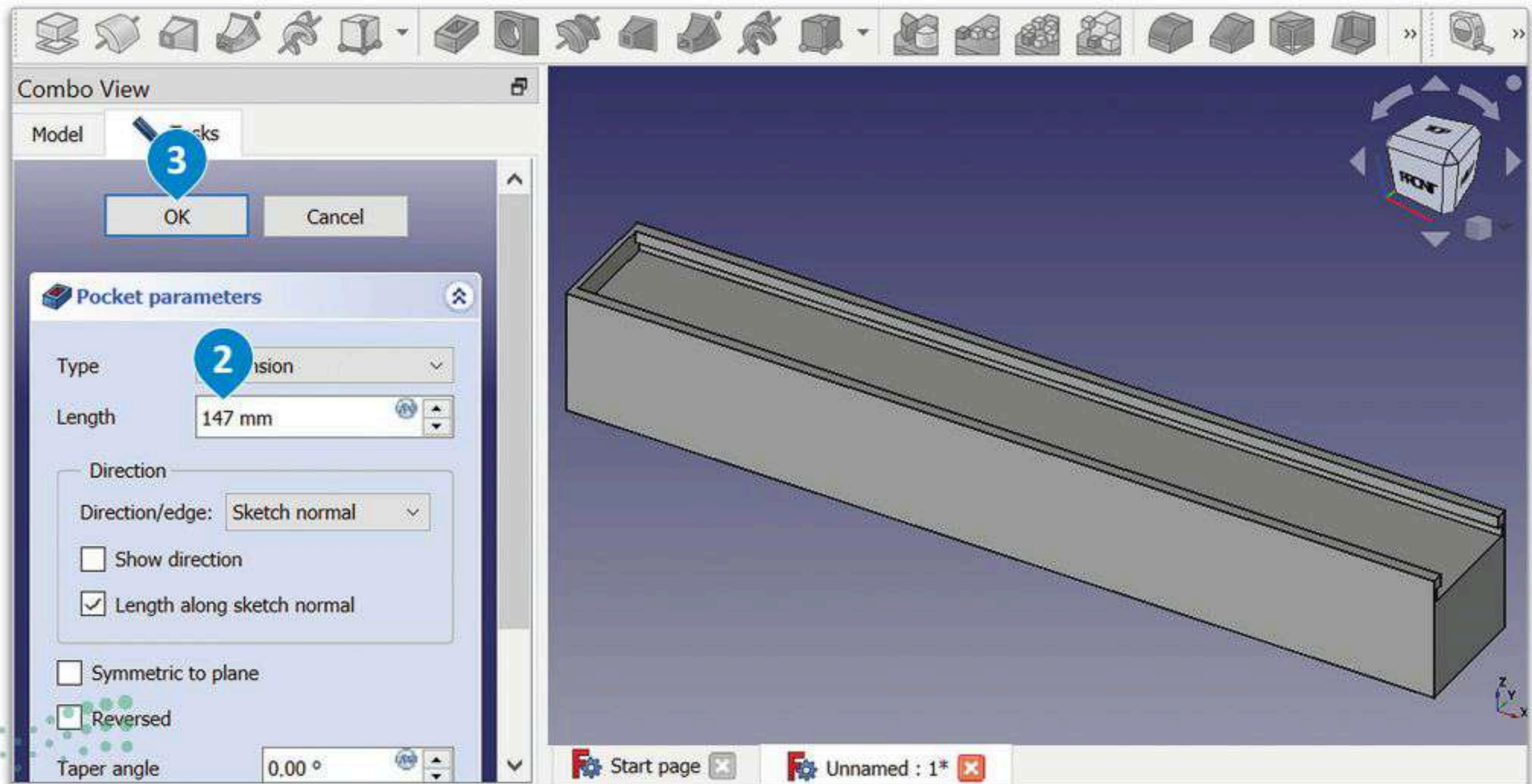
شكل 3.48: إنشاء التجويف
