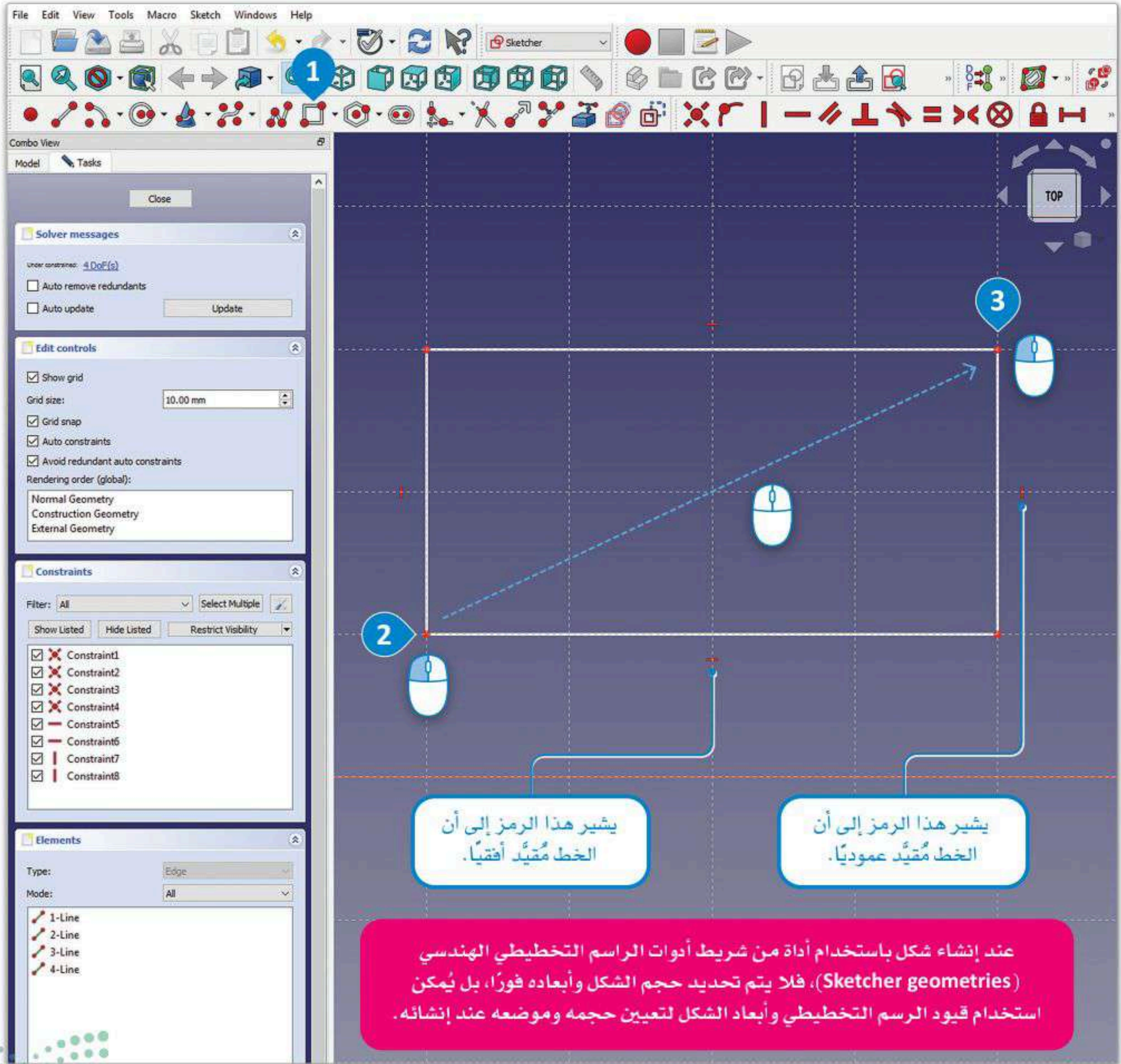
شكل 2.33: إنشاء مستطيل
