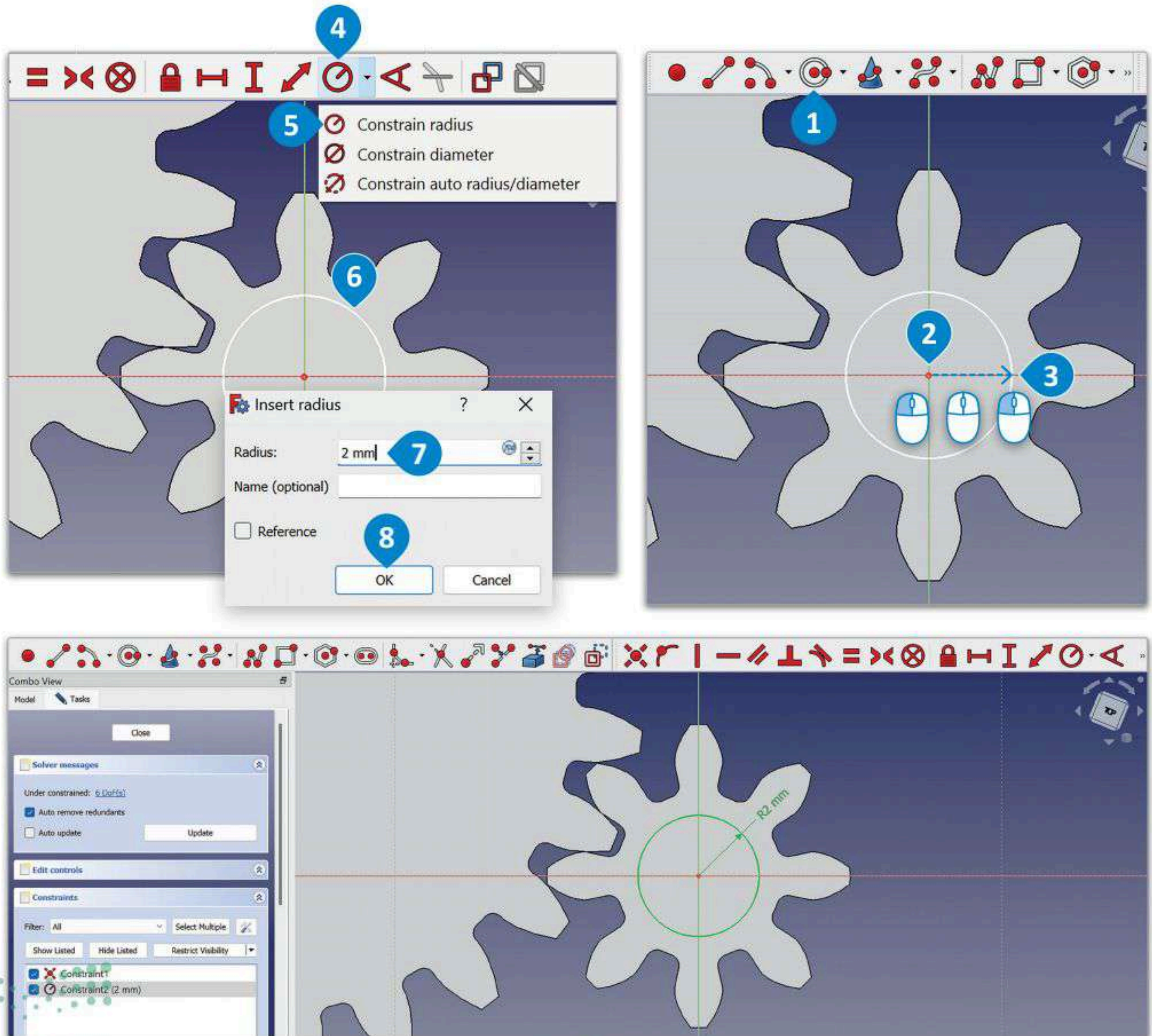
شكل 2.53: إنشاء دائرة
