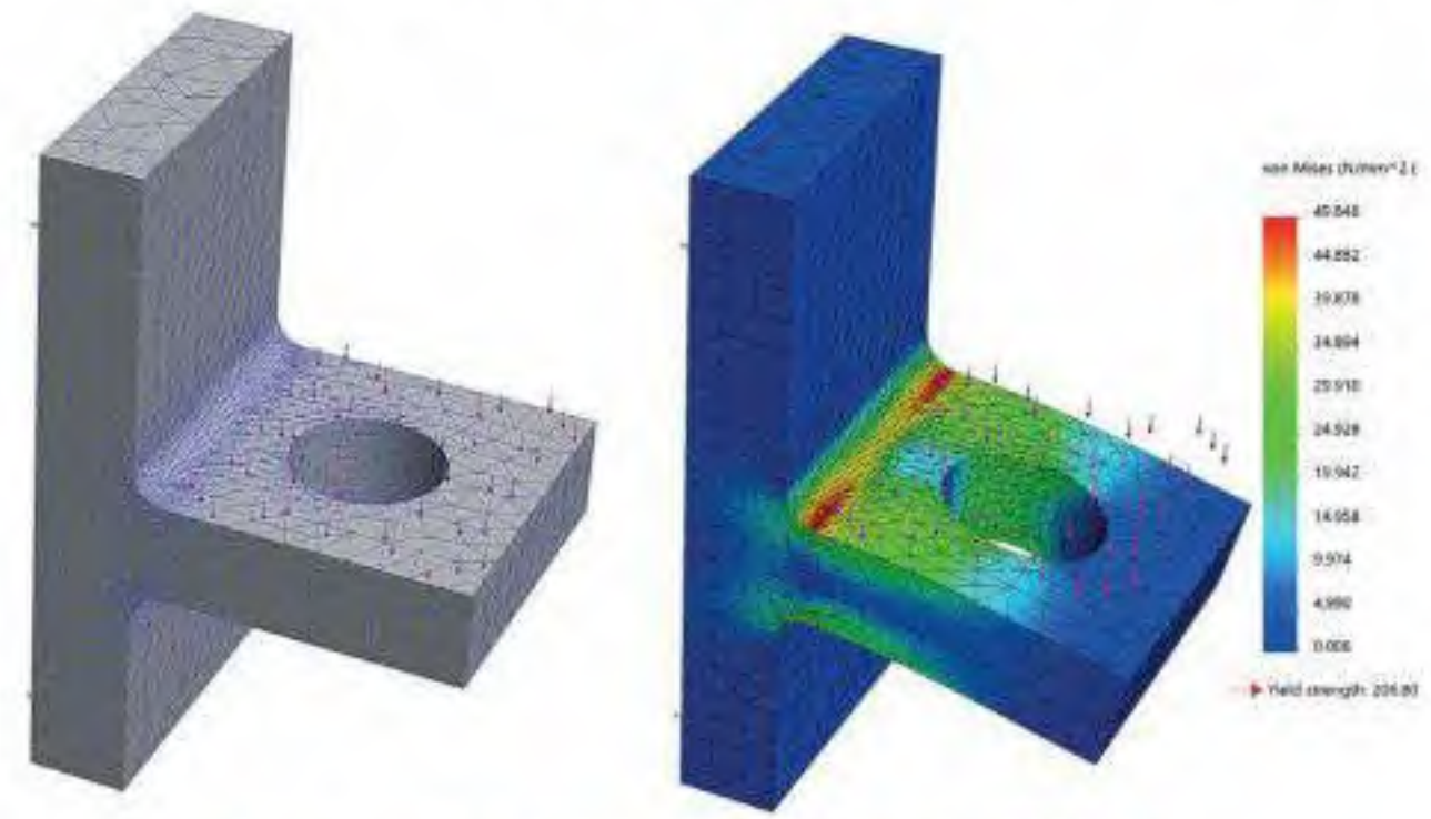
شكل 2.9: تحليل العناصر المحدودة ناتج عن نموذج صلب
