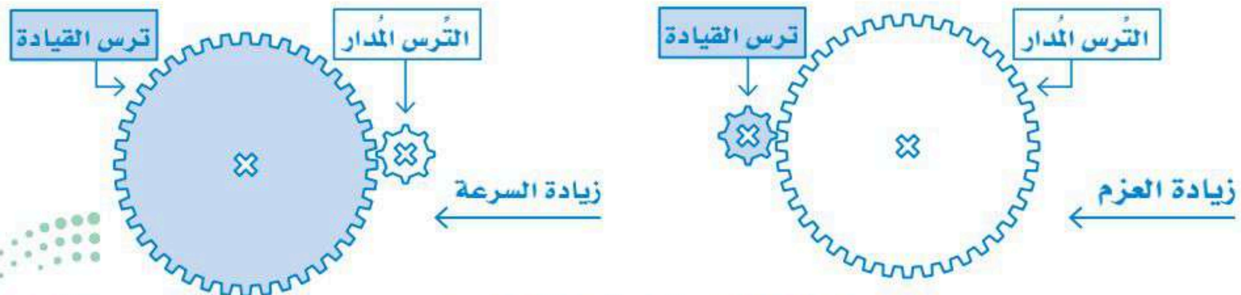
شكل 2.40: زيادة عزم الدوران مقابل زيادة السرعة
