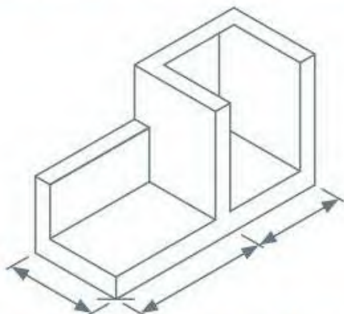
شكل 2.16: مثال على الرسم المتماثل القياس وزارة التعليم
