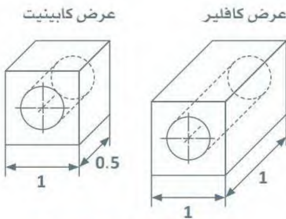
شكل 2.15: مثالان على الرسم الهندسي المائل
