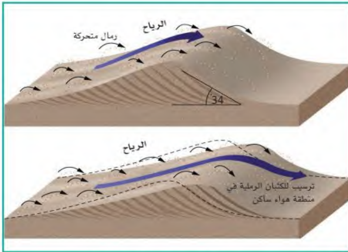
عملية تكوين الكتبان الرملية
