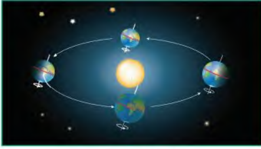
حركة الأرض حول الشمس
