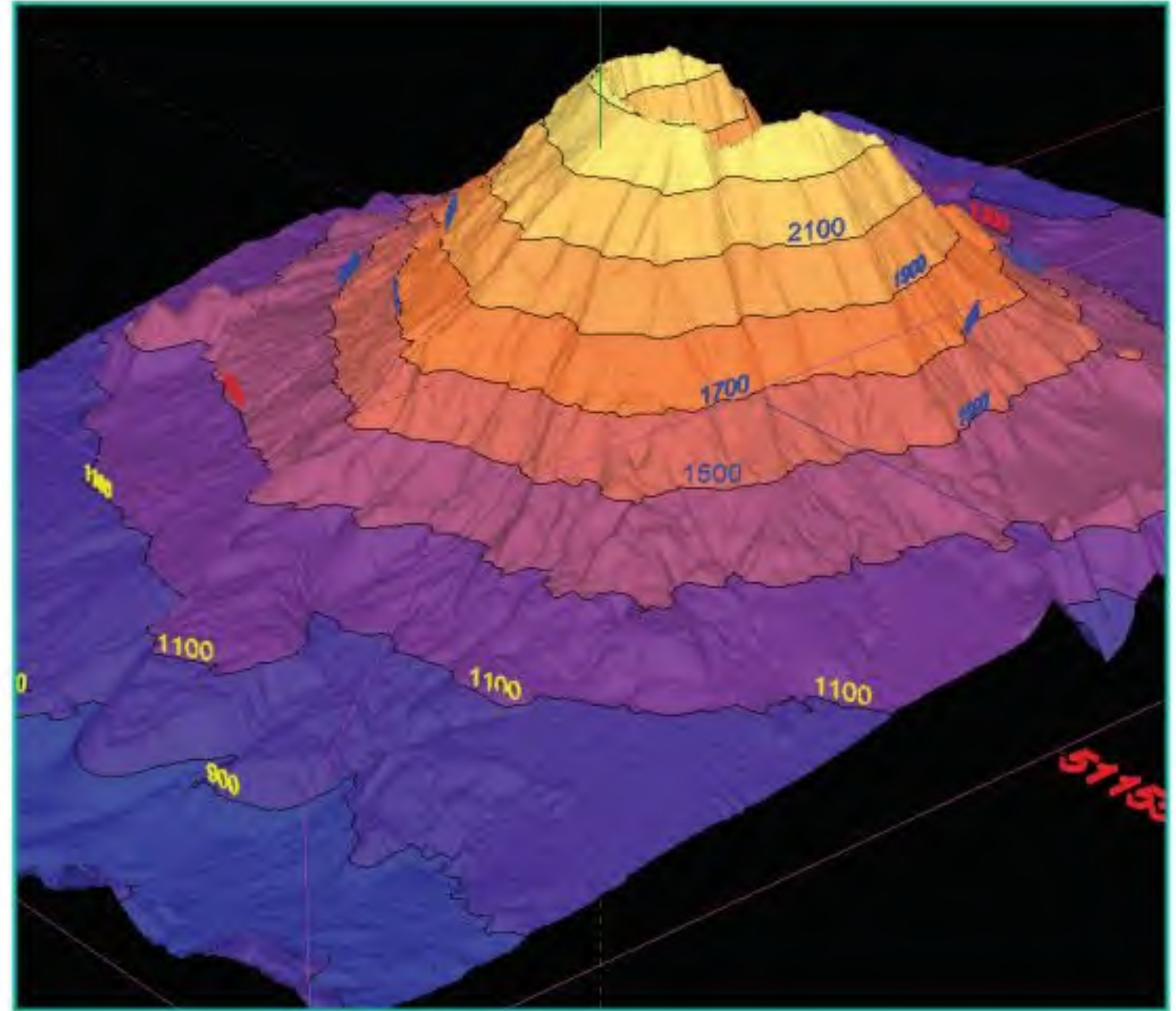
خطوط الكُنْتُور
