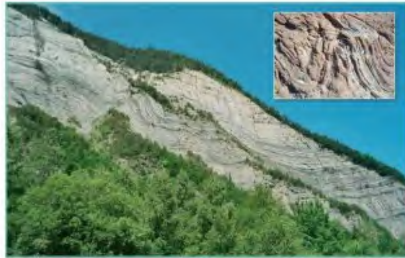
من أنواع الالتواءات
