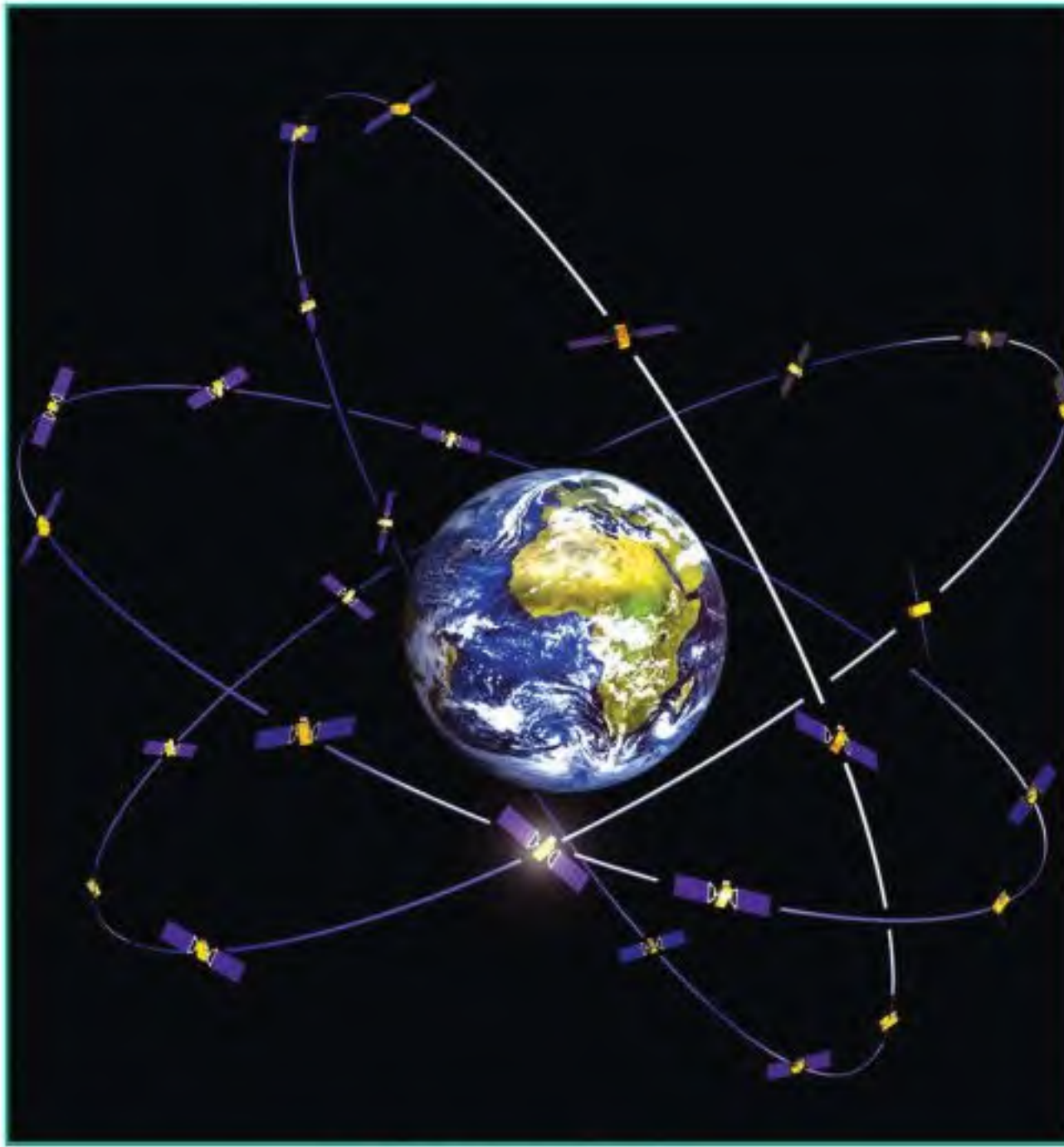
الأقمار الصناعية حول الأرض
