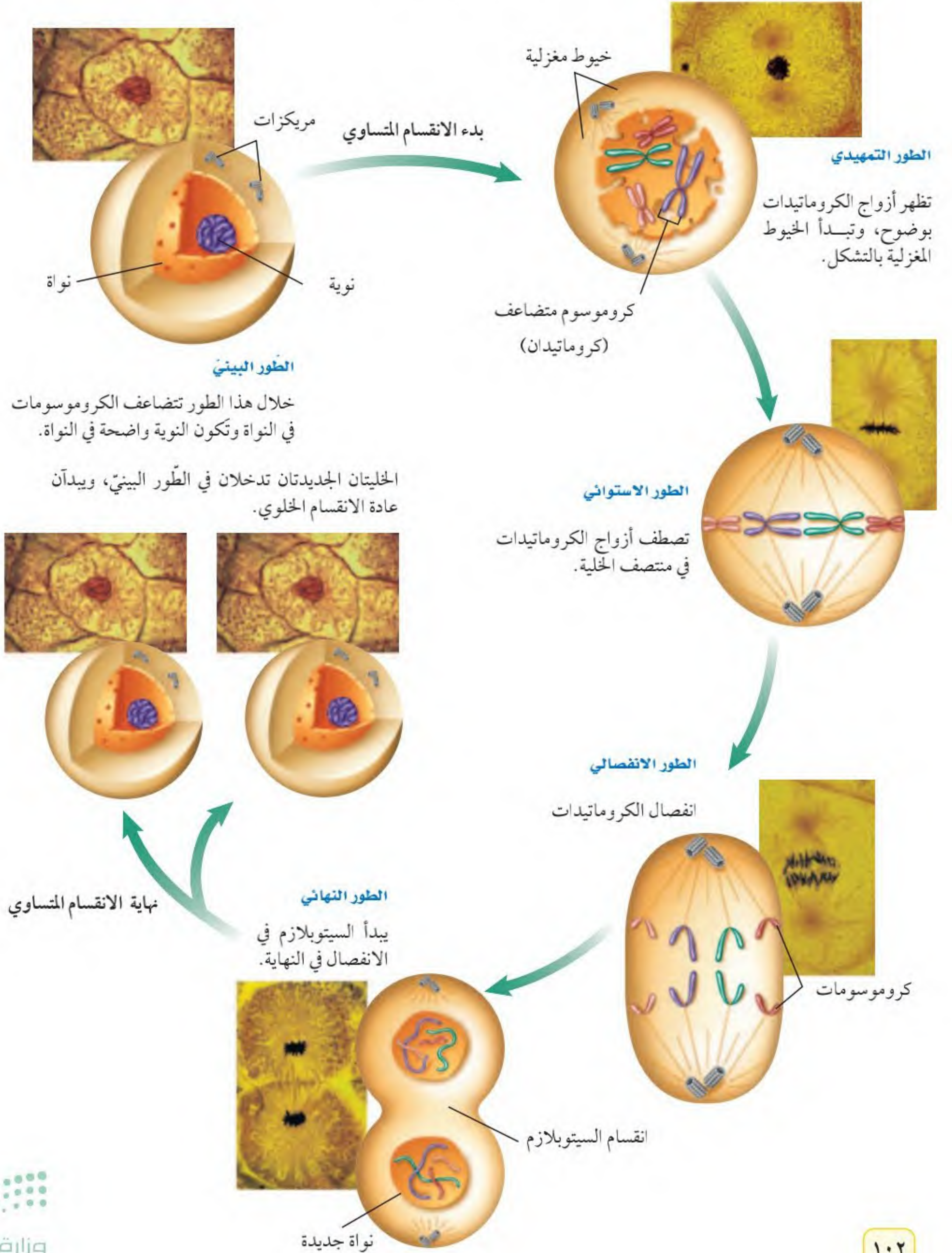
الشكل ١٦ يظهر الشكل الانقسام الخلوي لخلية حيوانية. الصور الظاهرة في الشكل مكبرة ٦٠٠ مرة.
