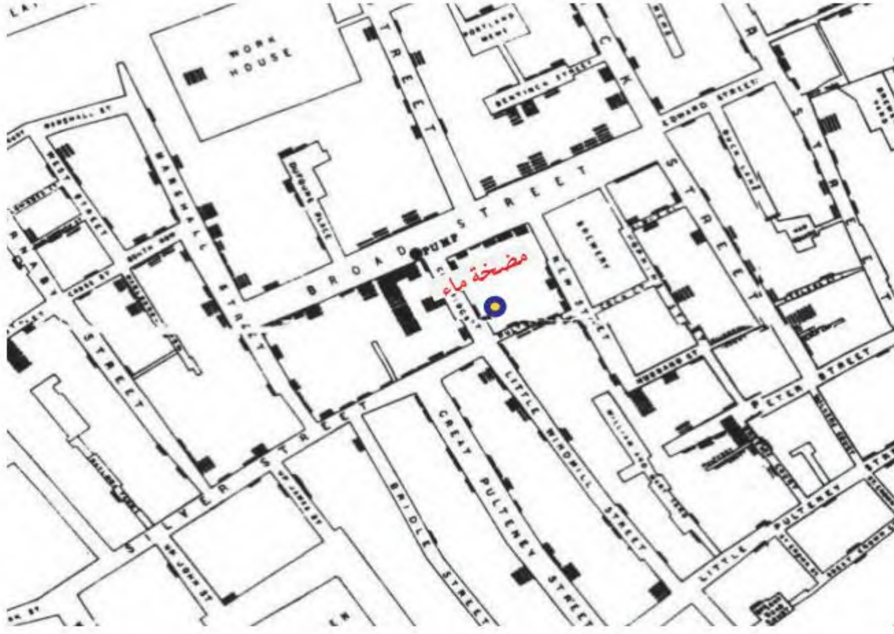
■ أماكن سكن المرضى المصابين بالكوليرا
