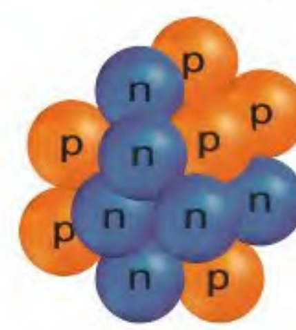
نواة ذرة كربون - ١٢
